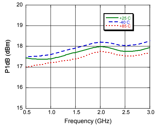
P1dB
