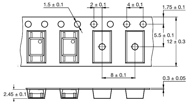
Fig. 17 - Tape Dimensions
