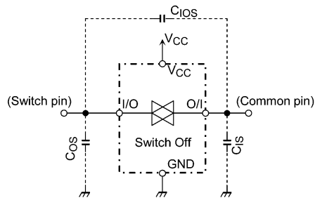
Figure 2 C_{1OS} , C_{1S} , C_{2S}
