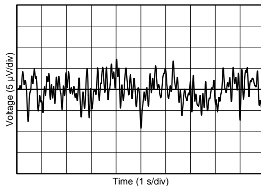
V_{BIAS} output
