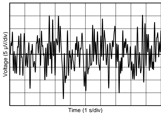
V_{REF} output
