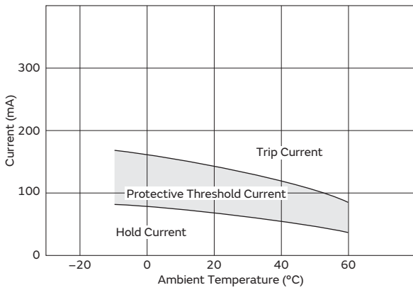
PTGL07BD330N3B51B0
