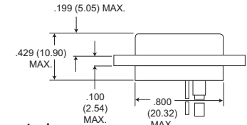
Receptacle
