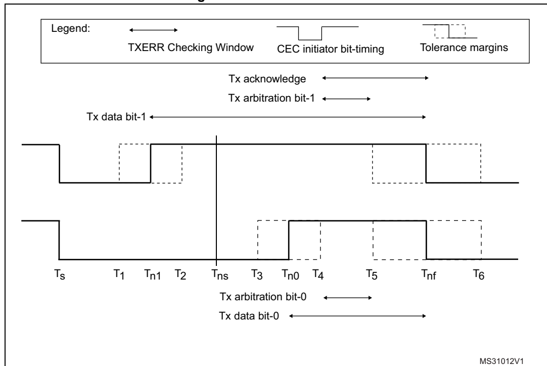
Figure 586. TXERR detection
