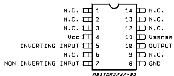
SO14
