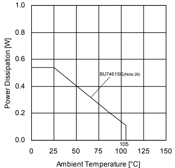
(d) BU7461SG
