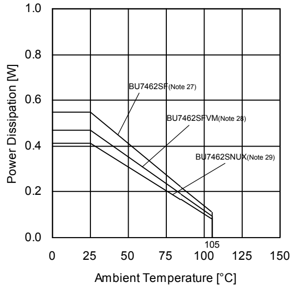
(f) BU7462Sxxx
