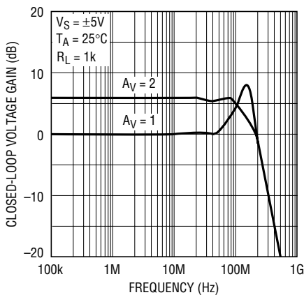
LT1191 • TA05
