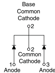
VS-30CTH02-1PbF
