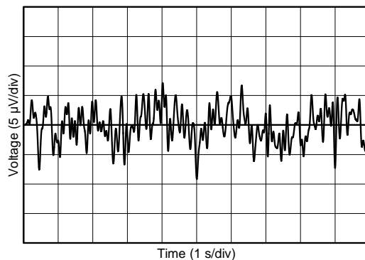
V_{BIAS} output
