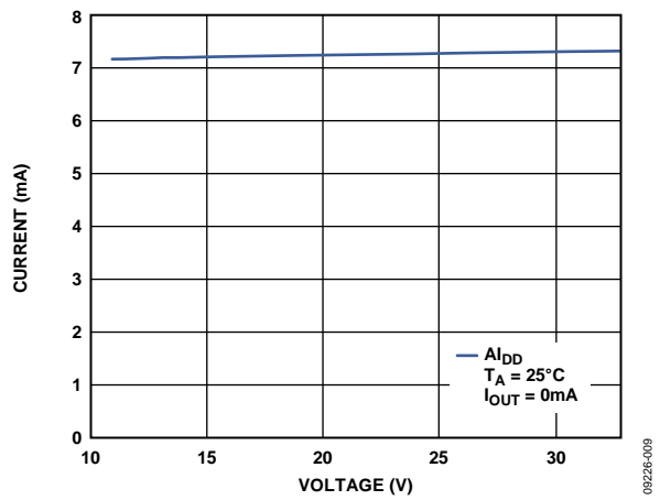
Figure 69. Al DD vs. AV DD
