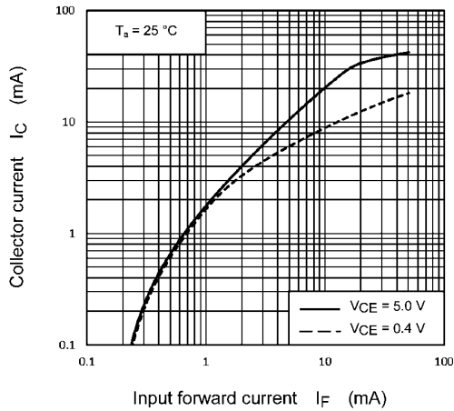
Fig. 11.9 I_C - I_F
