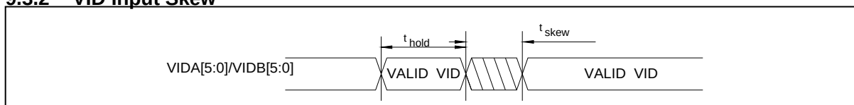
VID Input Timing
