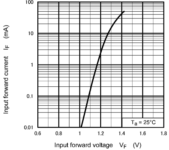
Fig. 11.4 I_F - V_F
