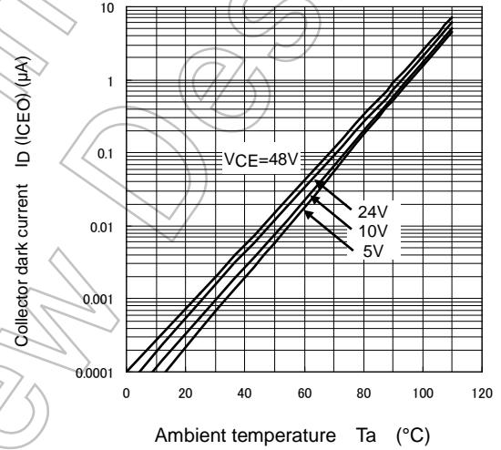
I_{CEO} - T_a
