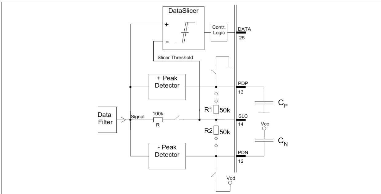
SLC_PkD.wmf
