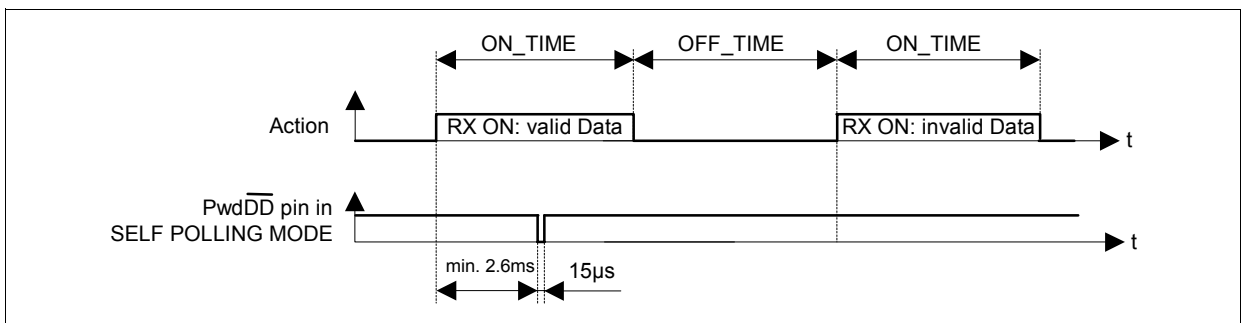
timing_selfpollmode.wmf
