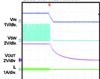
20ms/div.
