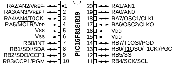
20-Pin SSOP
