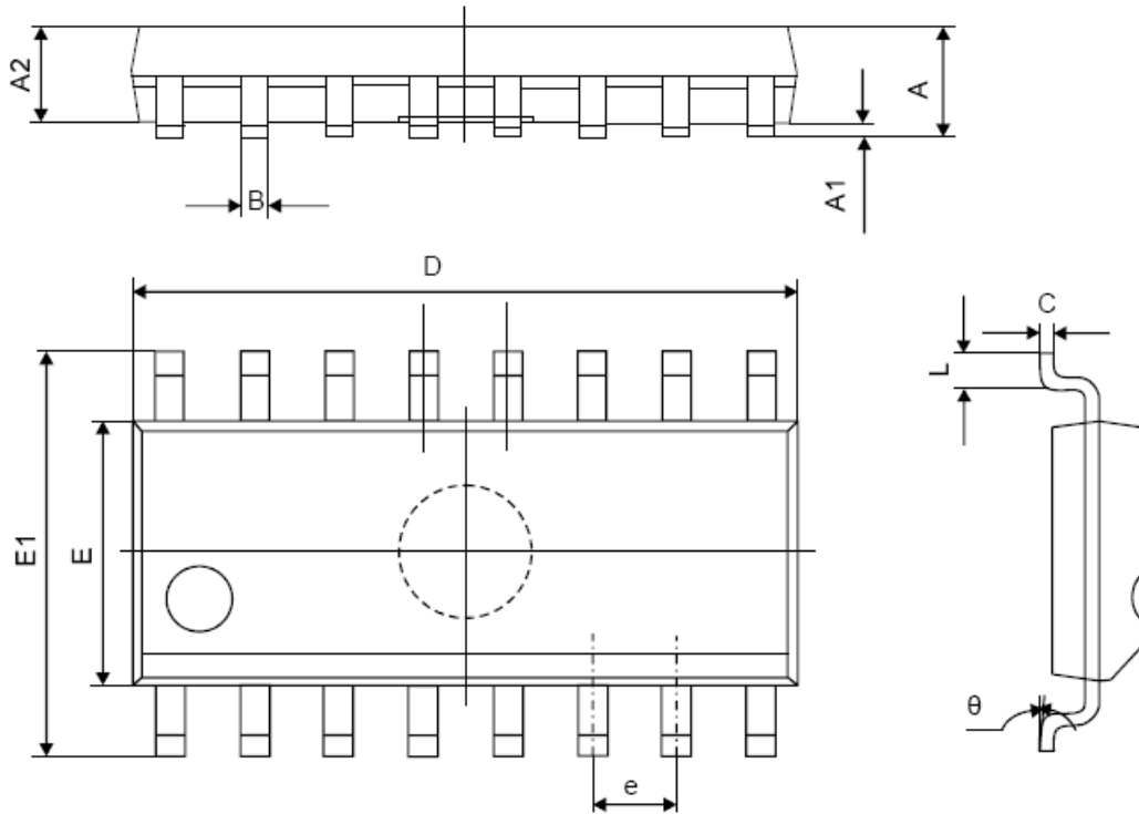
SOP-16
