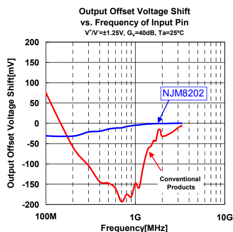
NJM8202RB1 (MSOP8(TVSP8))
