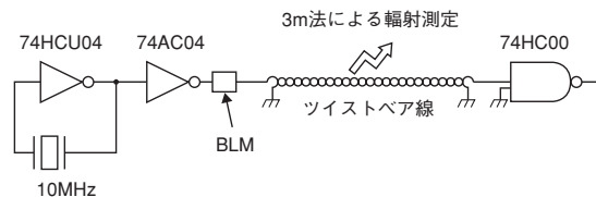
試験回路
