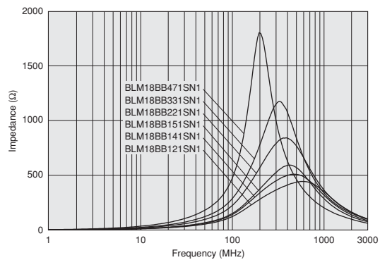
BLM18BBシリーズ (120Ω~470Ω)
