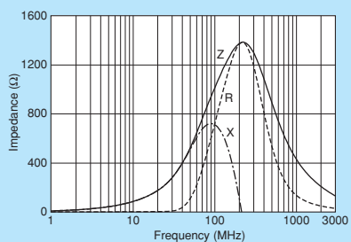
BLA2ABD102SN4
