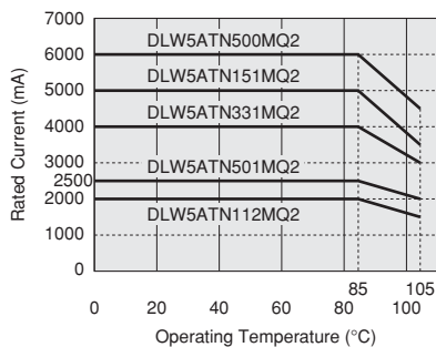
定格電流のディレーティング
