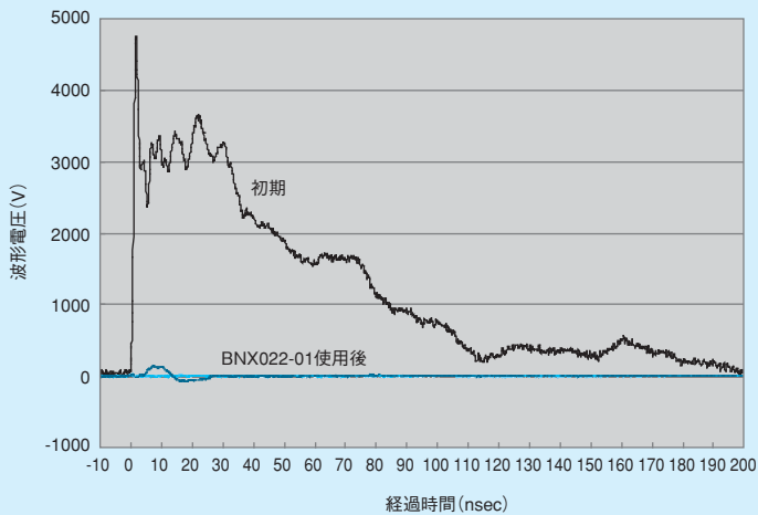
ESD波形比較
