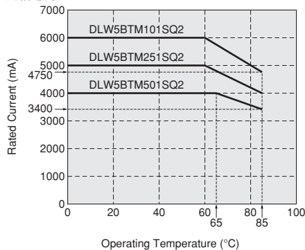
定格電流のディレーティング
