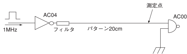
試験回路
