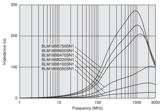
BLM18BBシリーズ (5Ω~75Ω)
