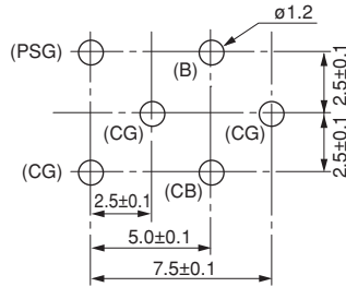
製品本体側の図
