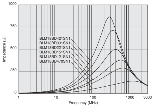
BLM18BDシリーズ (47Ω~420Ω)
