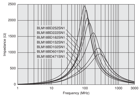
BLM18BDシリーズ (470Ω~2500Ω)
