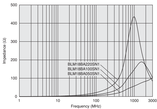
BLM18BAシリーズ (5Ω~22Ω)
