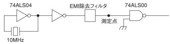
試験回路
