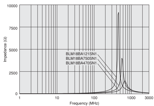
BLM18BAシリーズ (47Ω~120Ω)
