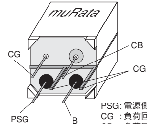
端子配列 (底面図)
