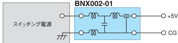
試験回路
