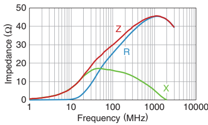
MPZ1005Y900CT000
