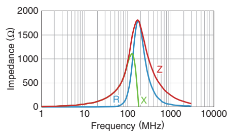
MMZ1608Q102BTA00
