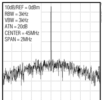
45MHz OUTPUT
