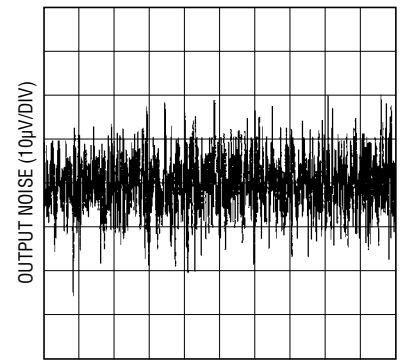
5V Output Noise 0.1\text{Hz} \leq f \leq 10\text{Hz}
