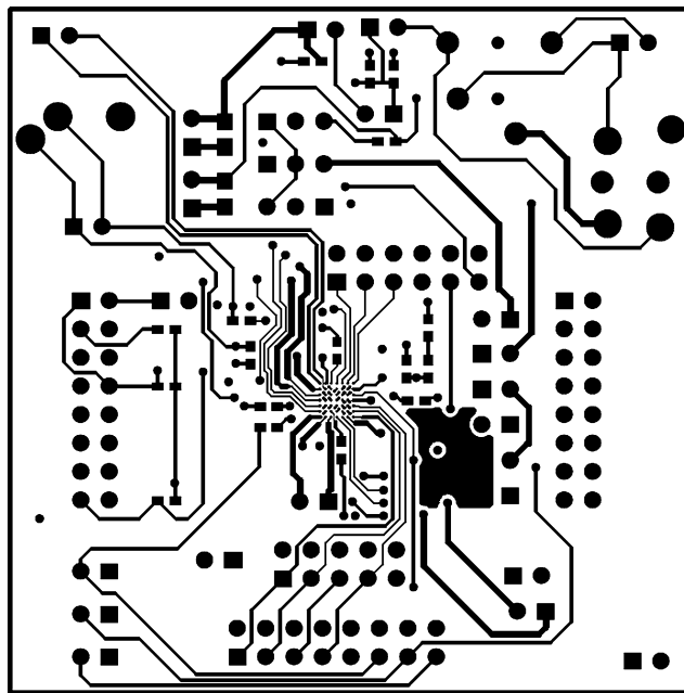
Figure 221. Top Layer
