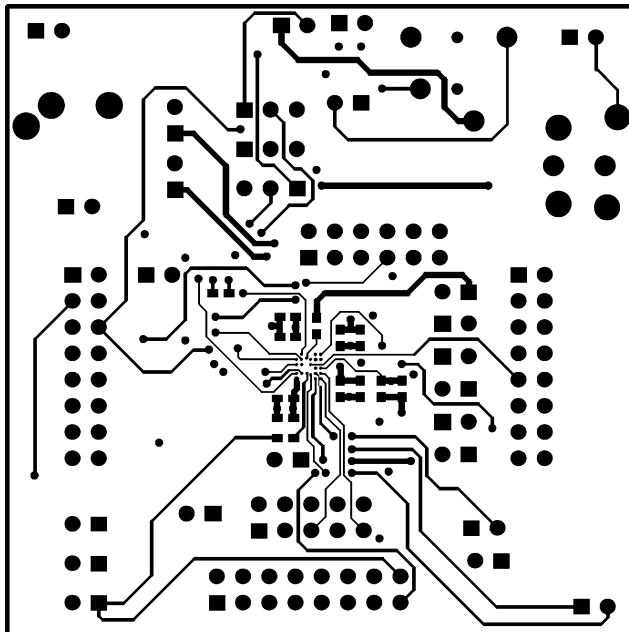
Figure 224. Bottom Layer
