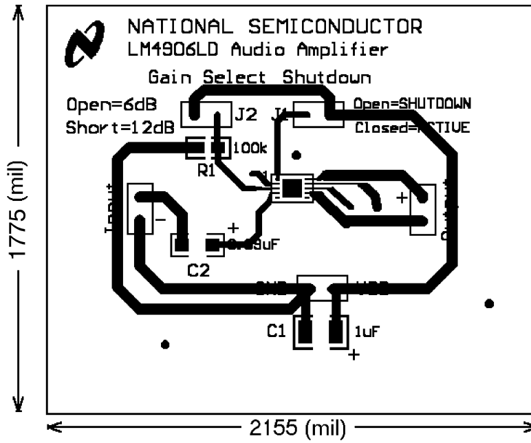
Figure 29. Top Layer
