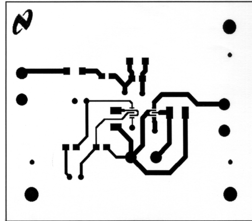
Top Layer
