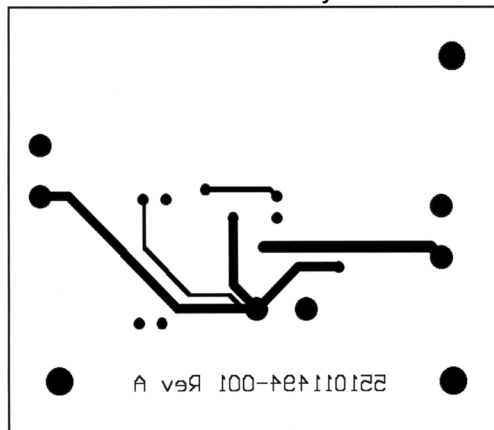
Bottom Layer
