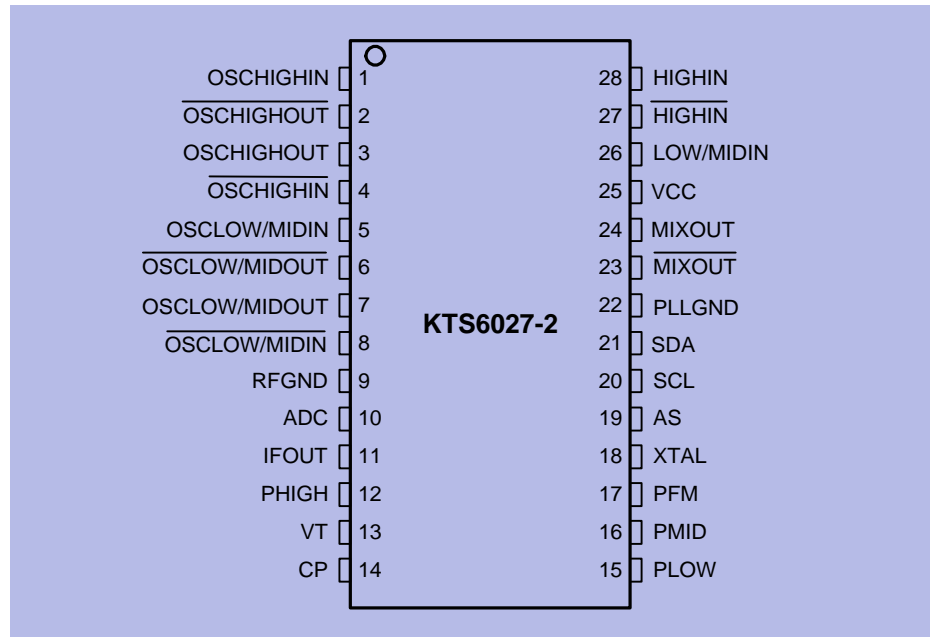
KTS6027-2_Pin_config
