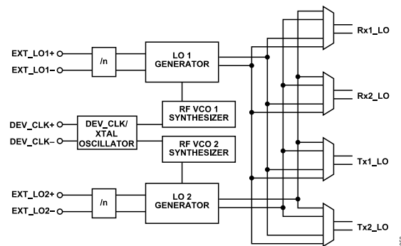
Figure 362. RF LO
