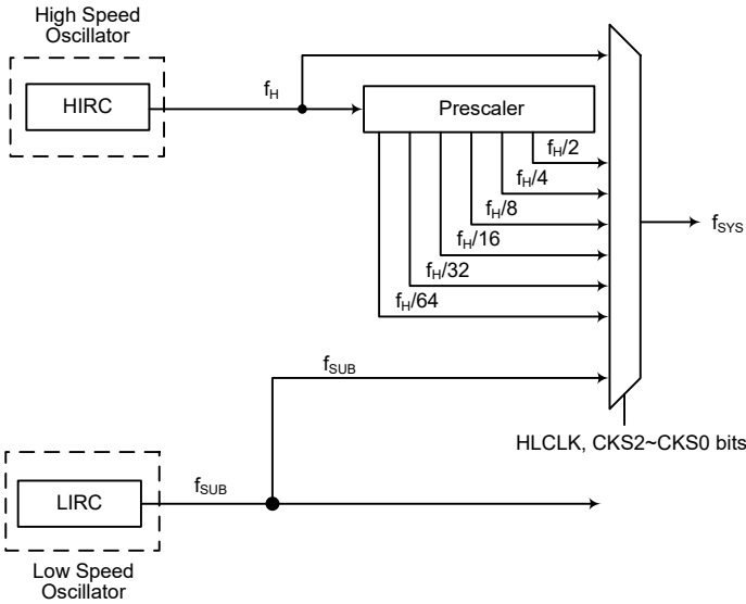
系统时钟配置
