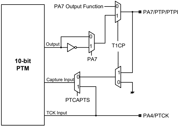
PTM 功能引脚控制方框图
