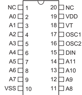
HT12F 20 SOP-A
