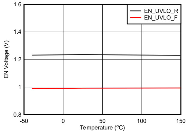
Figure 6-3. Enable UVLO
