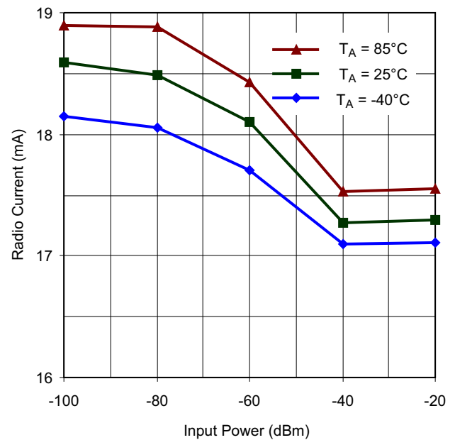
500 kBaud MSK
