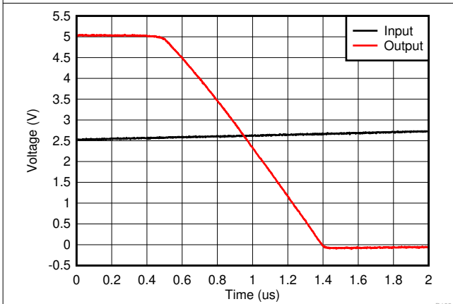
Figure 10-6. Falling Edge
