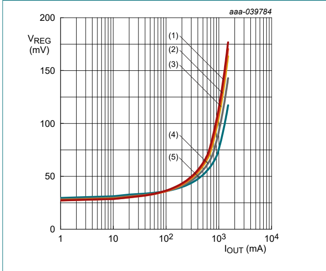
V_{IN} = 5 \text{ V}; V_{EN} = 0 \text{ V}; C_L = 100 \text{ nF} -40 °C 25 °C 85 °C 105 °C 125 °C (1) (2) (3) (4) (5)
