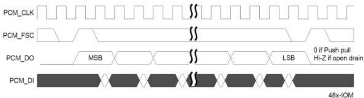
Figure 67. IOM format
