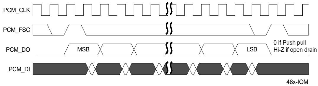
Figure 72: IOM format
