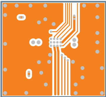
Figure 67: Mid layer 1 WLCSP
