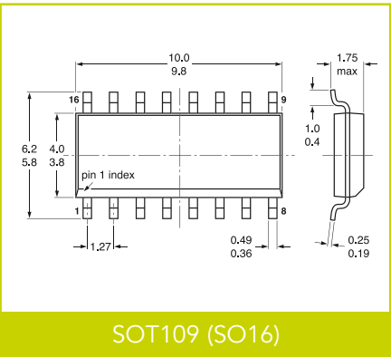
SOT109 (SO16)
