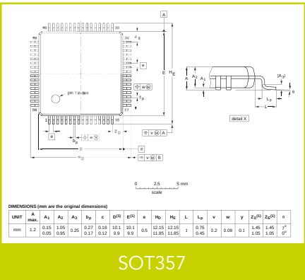
SOT357
