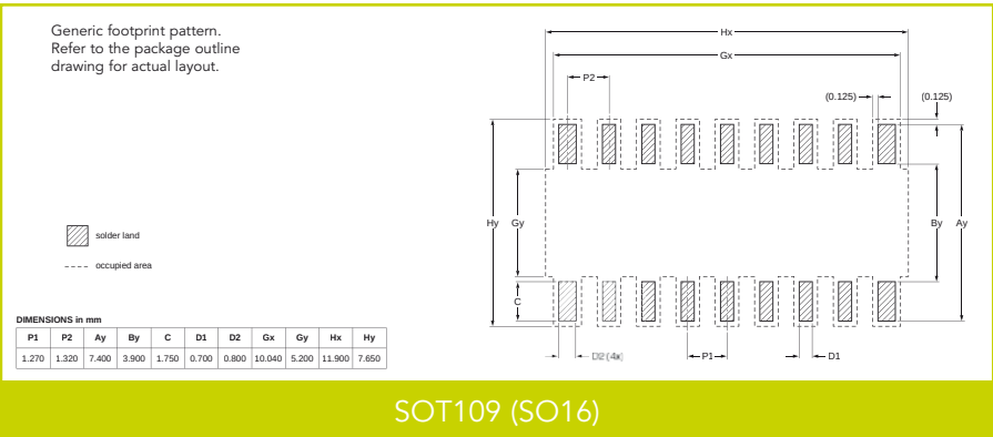
SOT109 (SO16)
