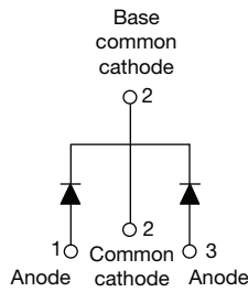
VS-30CTQ...-1-M3
