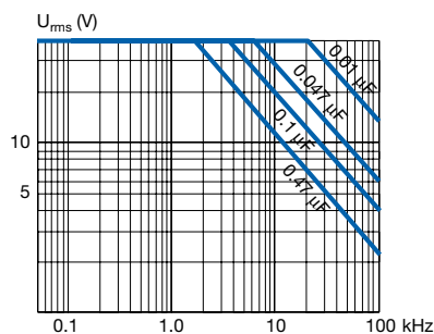
MMK5 63/40
