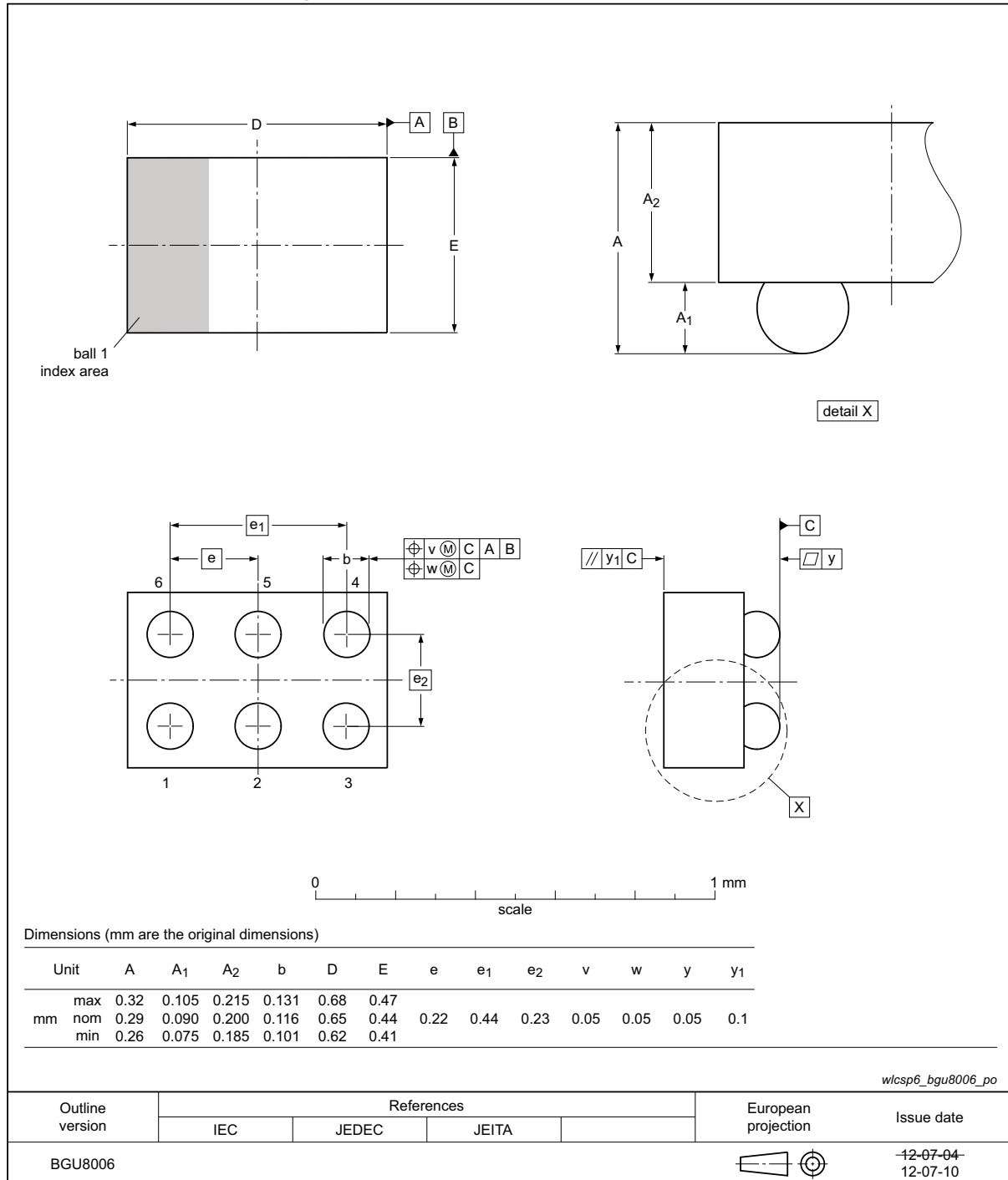
Fig 33. Package outline BGU8006 (WLCSP6)
