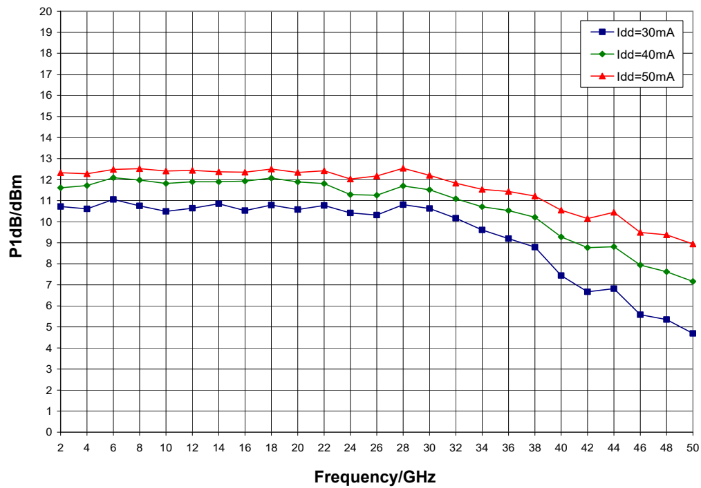
P1dB vs. I dd , V dd = 3 V, T A = 25 °C
