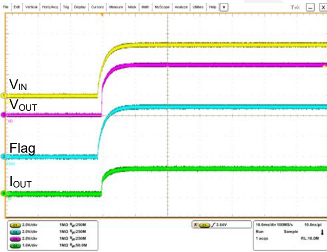
(EN = VIN, ROUT = 3.9 Ω, VIN = 0 ↑ 5V)
