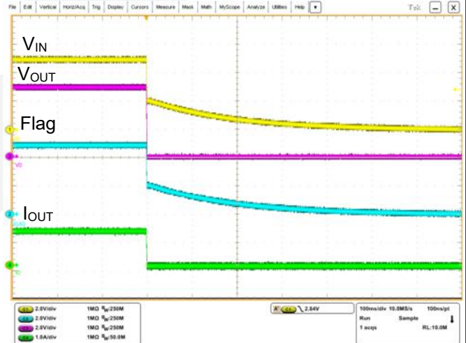
(EN = VIN, ROUT = 3.9 Ω, VIN = 5V ↓ 0)
