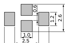
NFM31PC/31KC
