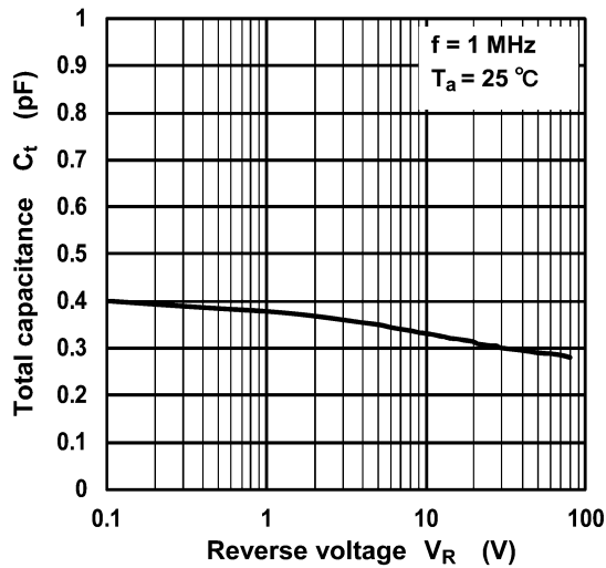
Fig. 8.3 C_t - V_R
